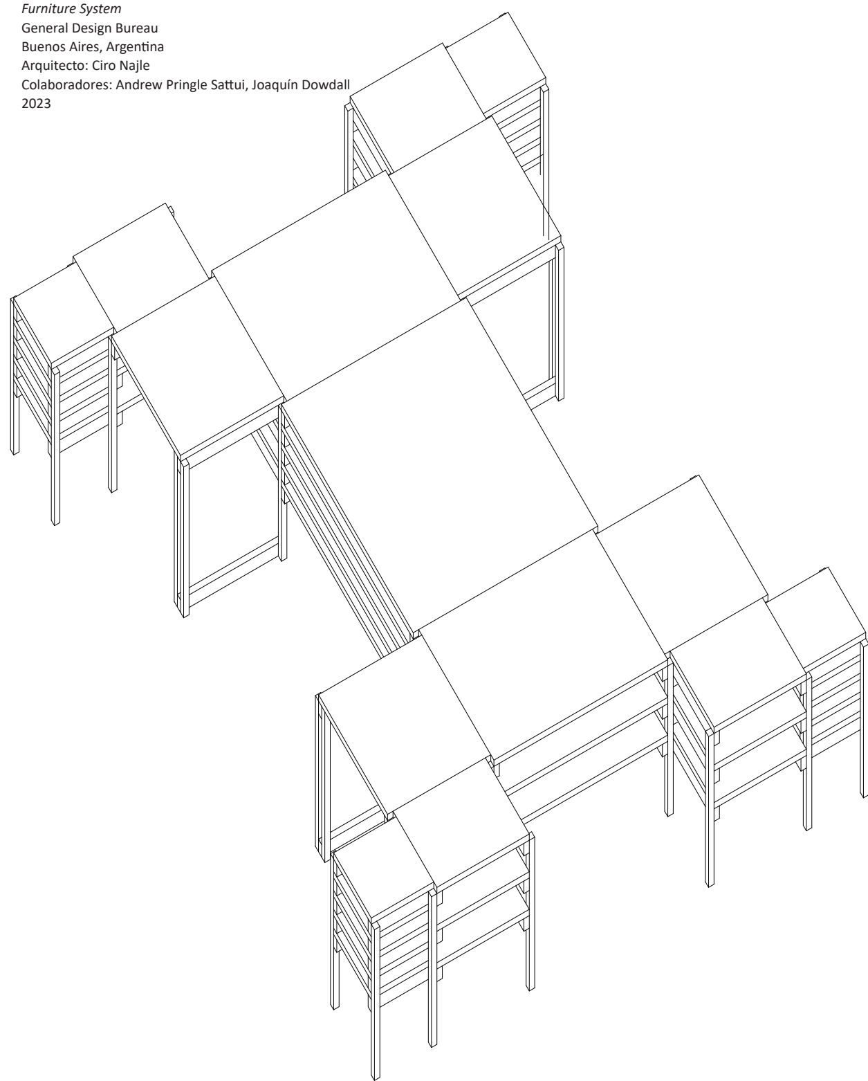
Escritoriolo seleccionado, variación de la subdivisión de la altura, escalonamiento e incremento de repisas con una tapa en la A2, 3 tapas cada 6 módulos en la A1 y A3, 5 tapas cada 3 módulos en la A0, y A4. Axonométrica. Escala 1.75.
