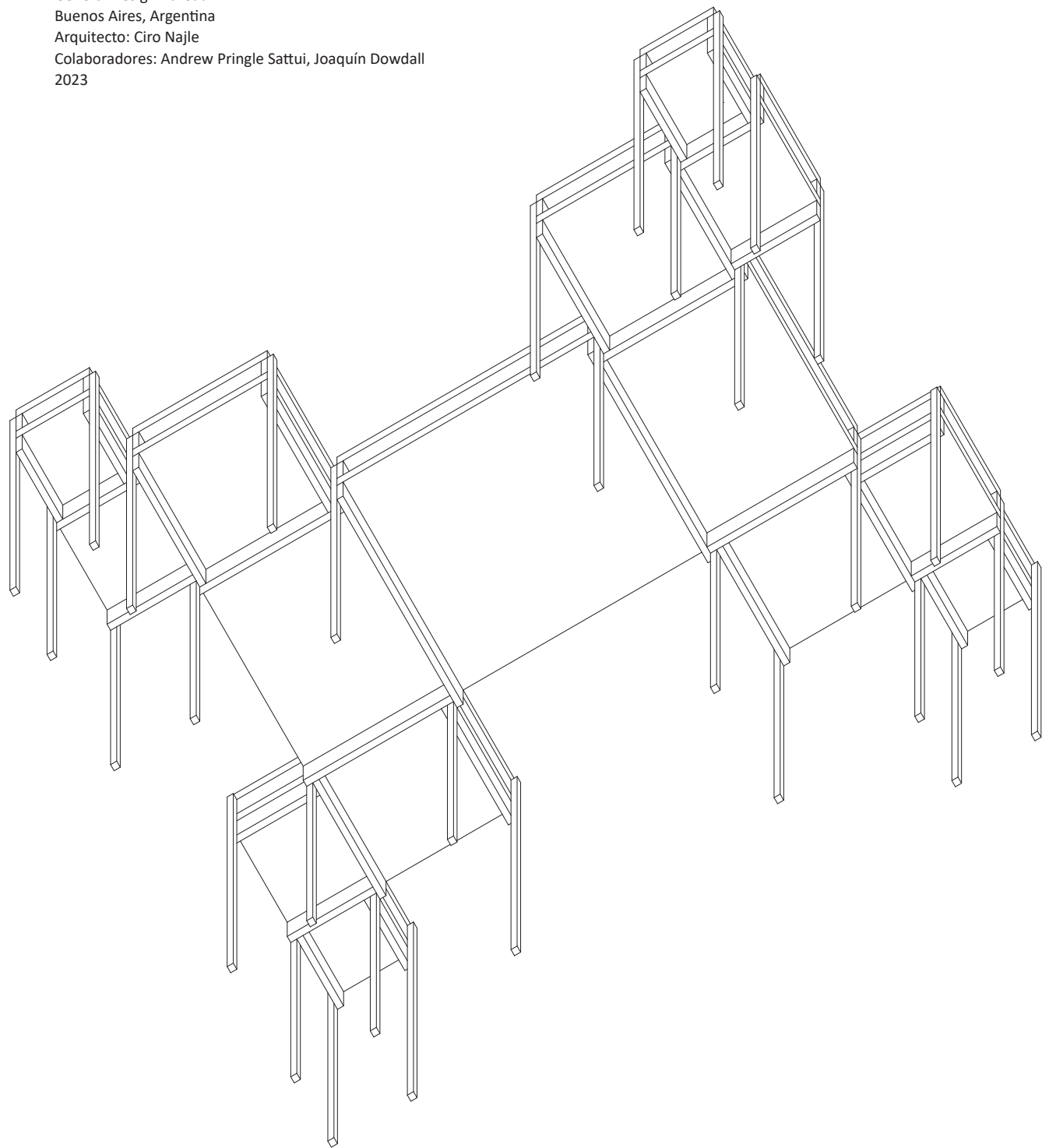
Escritoriolo Despacho Axonométrica inferior 135 grados. Escala 1.25.
