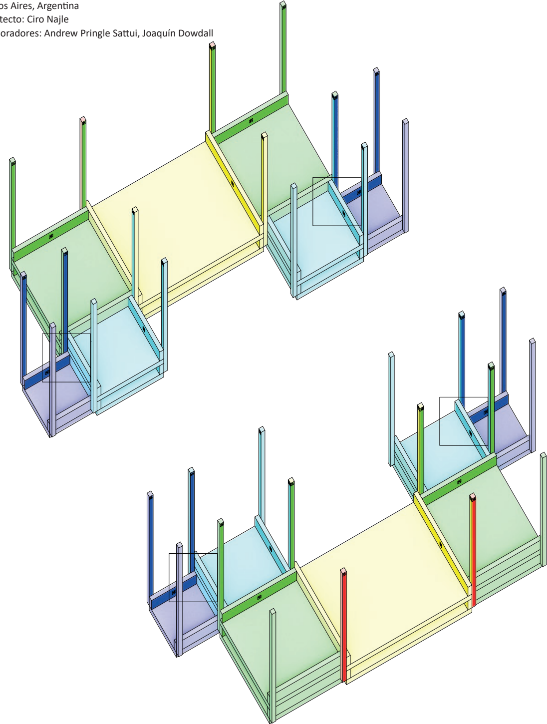
Escritoriolo Despacho. Axonometría. Escala 1:25. 25 Unir las bandejas A3 con patas a las bandejas A2 con patas, de manera que las patas de la A4 complementen a las A3
