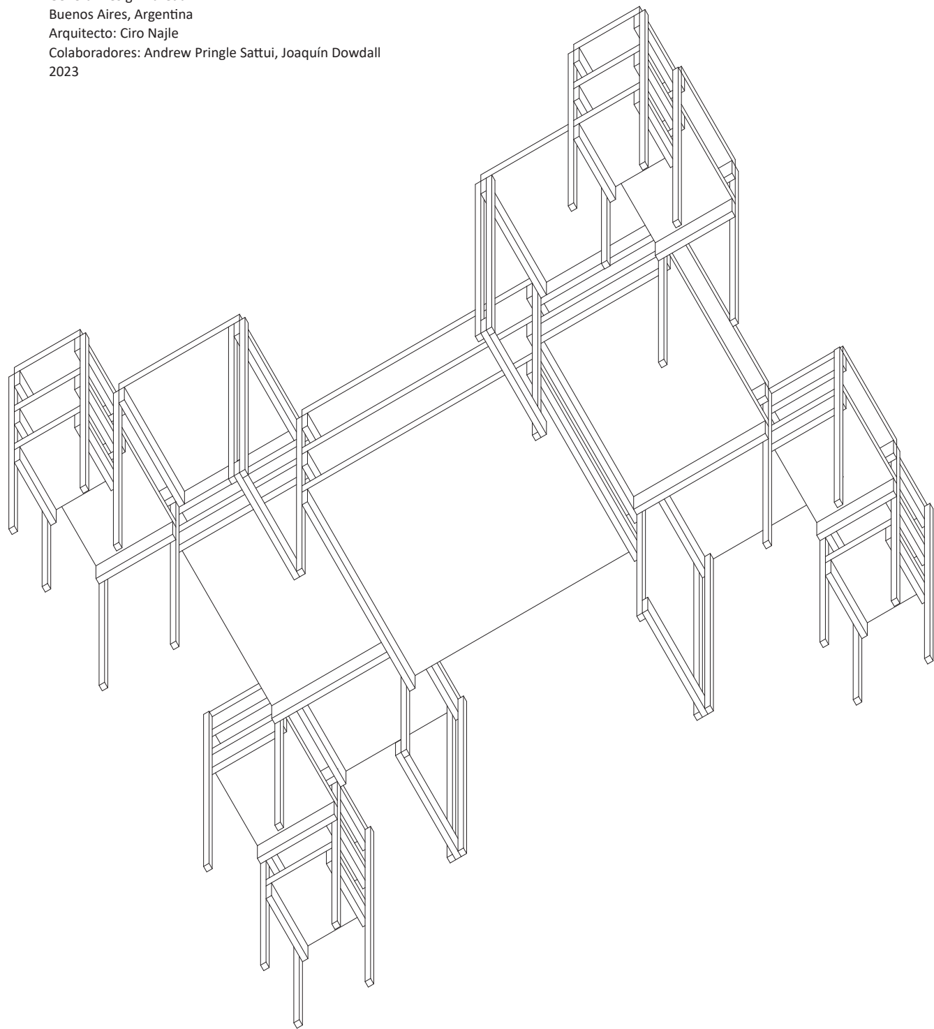
Escritoriolo Oficina Axonométrica inferior 135 grados. Escala 1.25.
