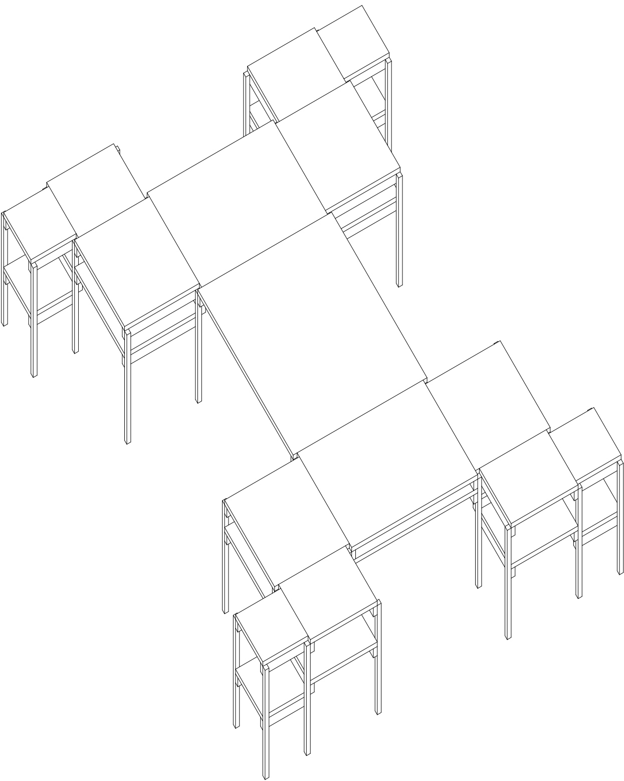
Escritoriolo seleccionado, variación de la subdivisión de la altura, con una repisa inferior escalonada de la tapa superior de la A0 a la mitad de la altura de la A4. Axonométrica. Escala 1.75.
