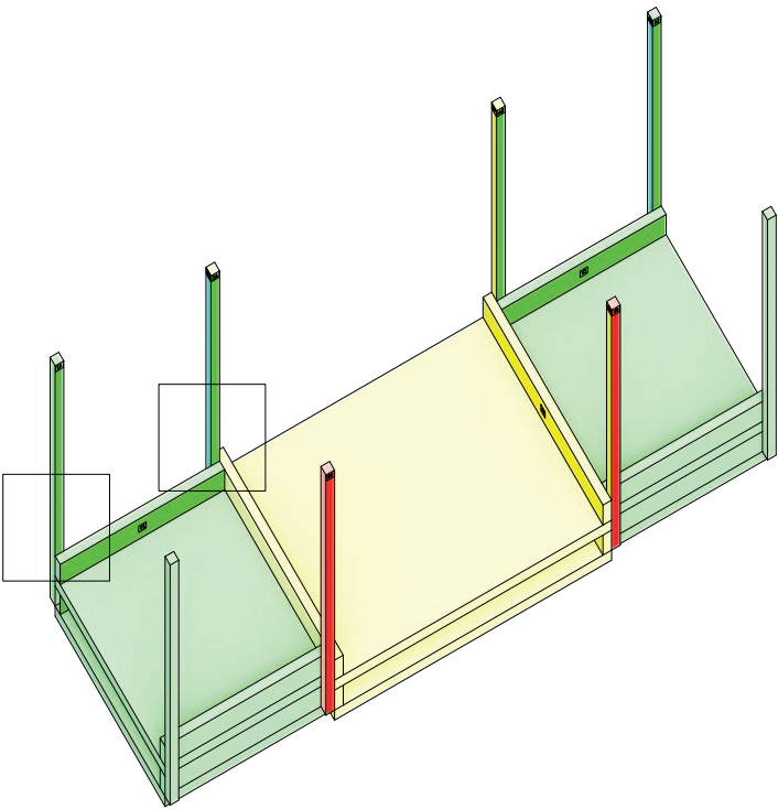
Escritoriolo Despacho. Axonometría. Escala 1:25. 12 Apoyar las cuatro bandejas A2 restantes sobre las bandejas A2 ya unidas a las patas 13 Unir las cuatro bandejas apoyadas con sus respectivas cuatro patas
