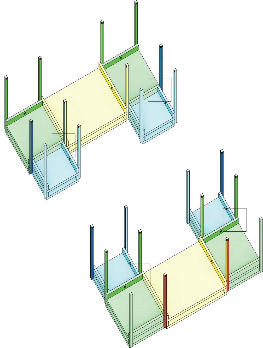
Escritoriolo Despacho. Axonometría. Escala 1:25. 19 Apoyar las cuatro bandejas A3 restantes sobre los tacos de 18cm 20 Unir las cuatro bandejas apoyadas con sus respectivas cuatro patas
