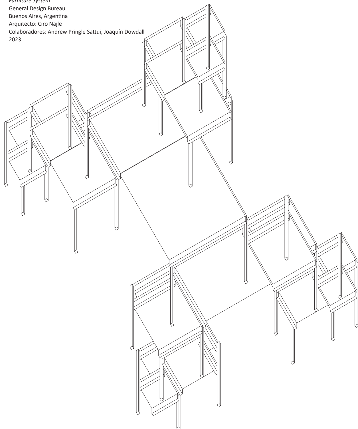
Escritoriolo Taller Axonométrica inferior 045 grados. Escala 1.25.
