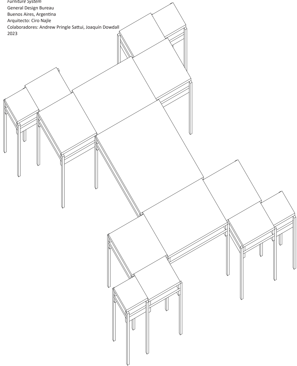
Escritoriolo seleccionado, variación de la subdivisión de la altura, con una repisa inferior a la misma altura. Axonométrica. Escala 1.75.
