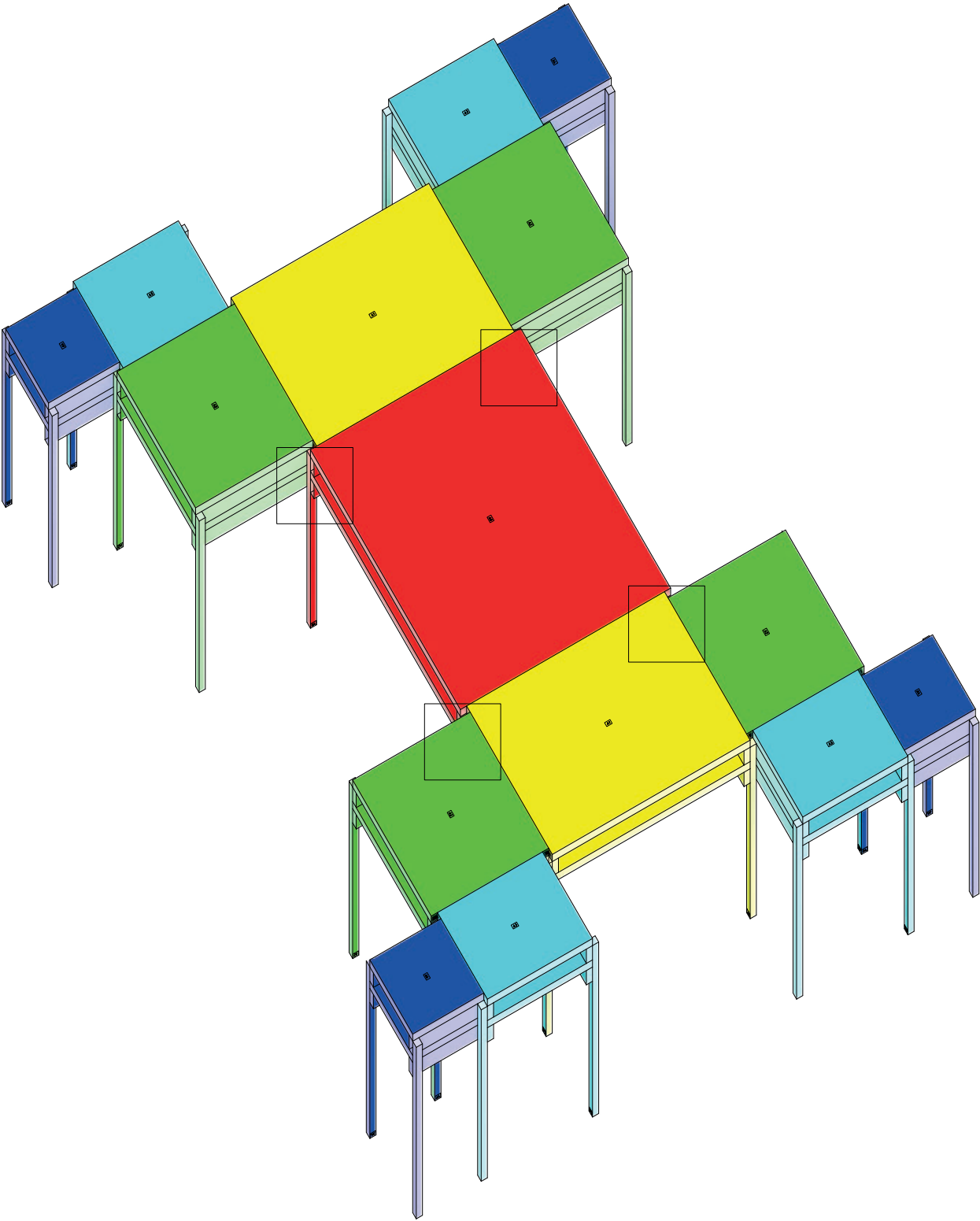
Escritoriolo Despacho. Axonometría. Escala 1:25. 31 Unir la siguiente bandeja A0 con las dos mitades de manera de puntearlas
