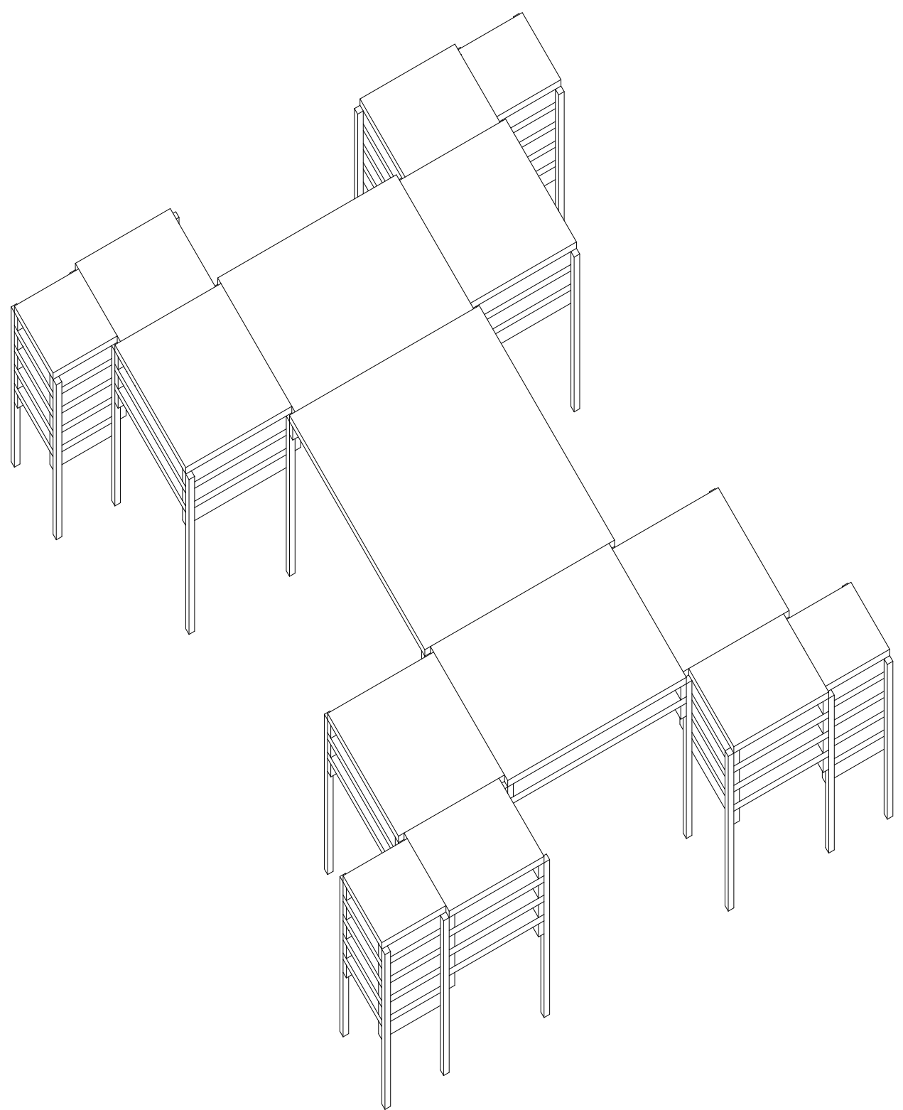
Escritorio seleccionado, variación de la subdivisión de la altura, escalonamiento e incremento de repisas cada 3 modulos con una tapa en la A0 a 5 tapas en la A4. Axonométrica. Escala 1.75.
