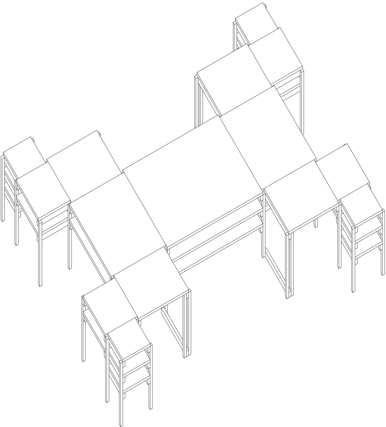
Escritoriolo Oficina Axonométrica superior 135 grados. Escala 1.25.
