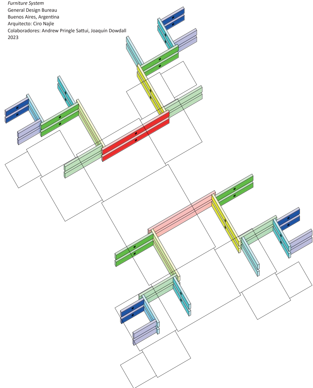
Escritoriolo Despacho Axonometría. Vigas. Escala 1:25
