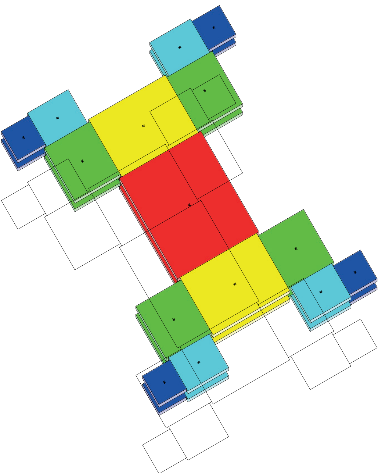
Escritoriolo Despacho Axonometría. Tablas. Escala 1:25
