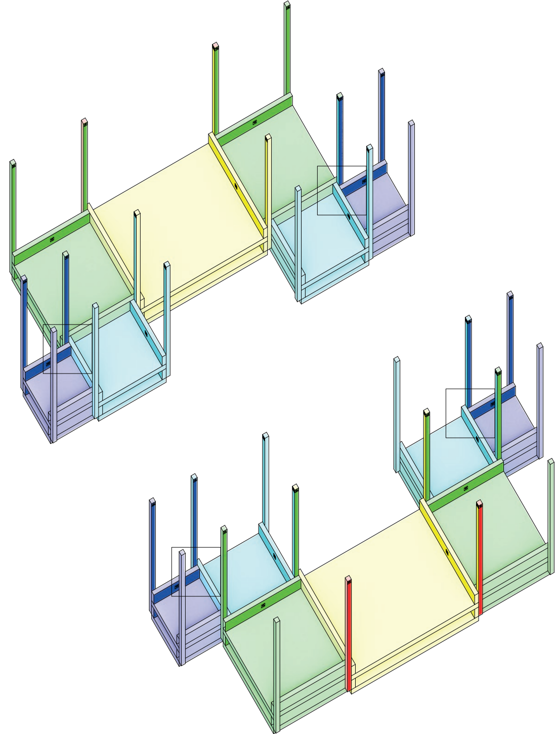
Escritoriolo Despacho. Axonometría. Escala 1:25. 26 Apoyar las cuatro bandejas A4 restantes sobre los tacos de 27cm 27 Unir las cuatro bandejas apoyadas con sus respectivas cuatro patas
