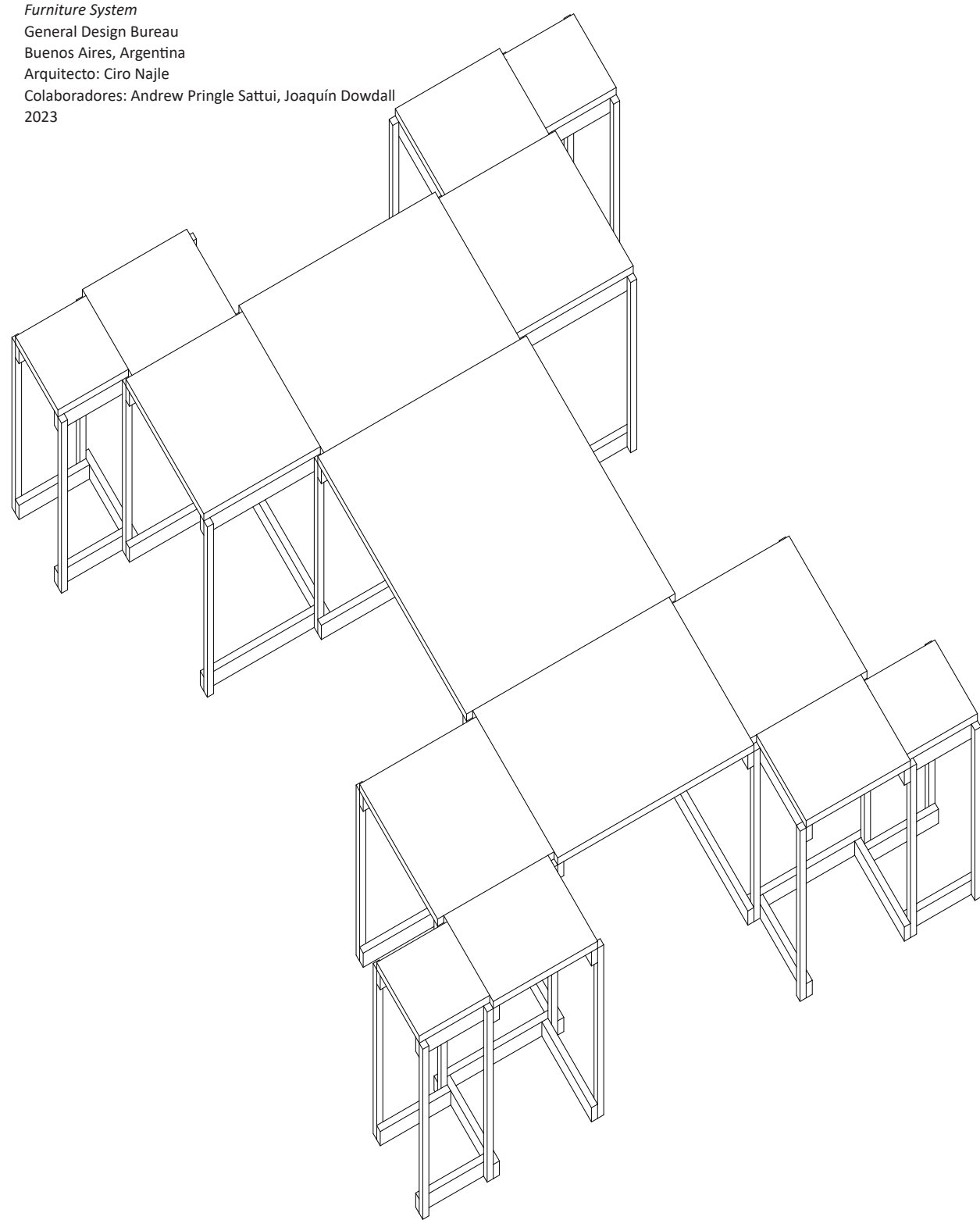
Escritoriolo seleccionado, variación de la subdivisión de la altura, sin subdivisión con vigas inferiores. Axonométrica. Escala 1.75.
