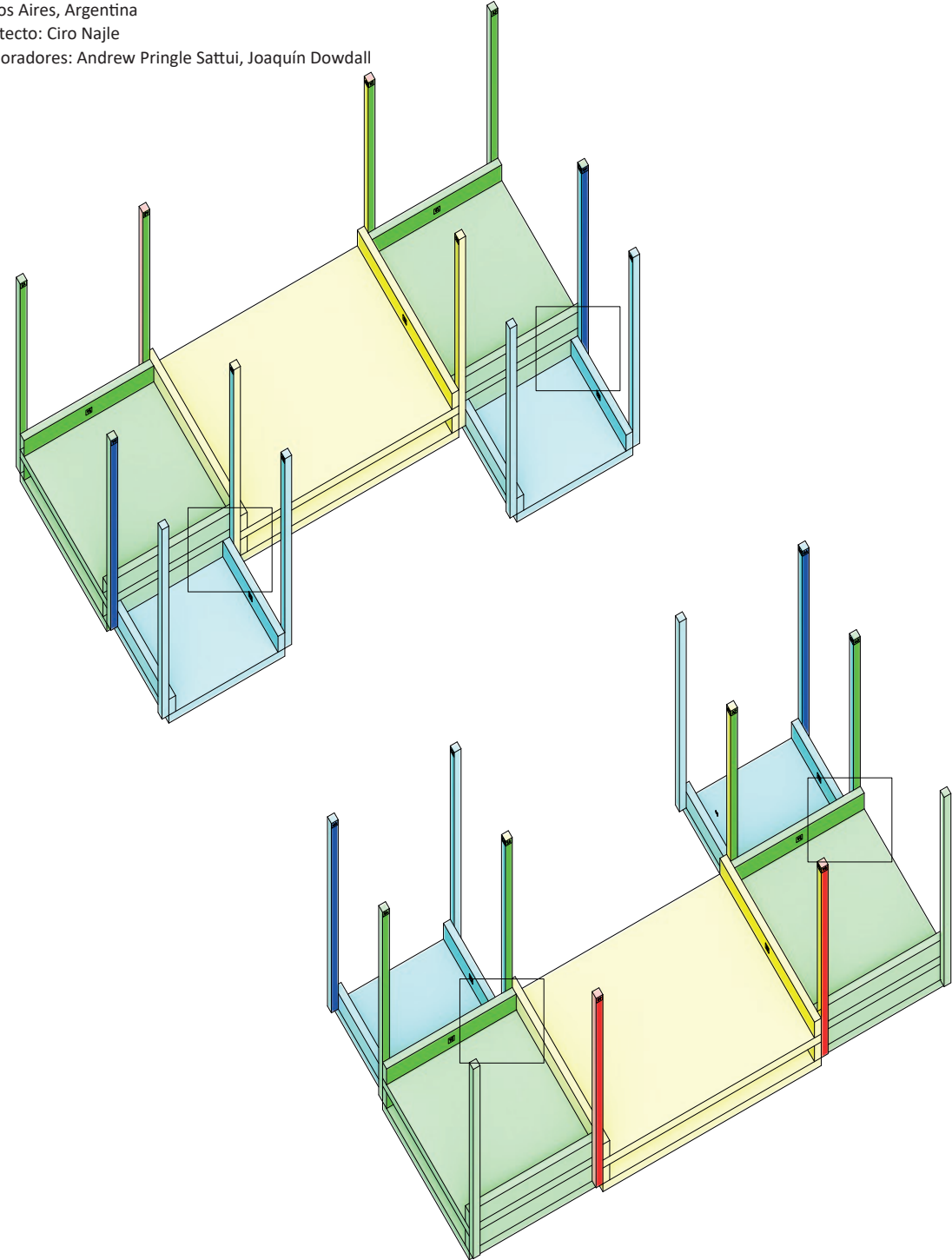
Escritoriolo Despacho. Axonometría. Escala 1:25. 18 Unir las bandejas A3 con patas a las bandejas A2 con patas, de manera que las patas de la A3 complementen a las A2
