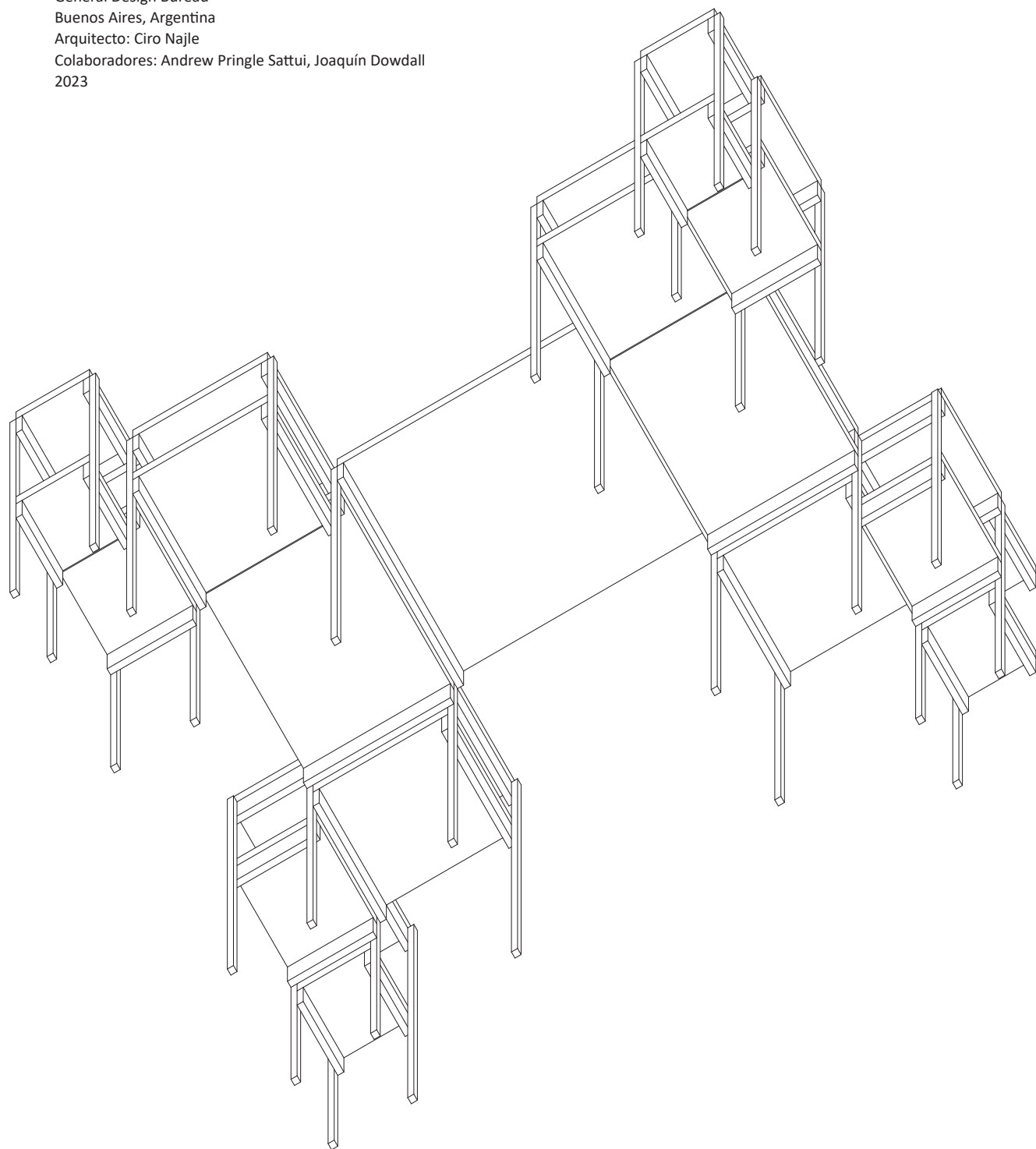
Escritoriolo Taller Axonométrica inferior 135 grados. Escala 1.25.
