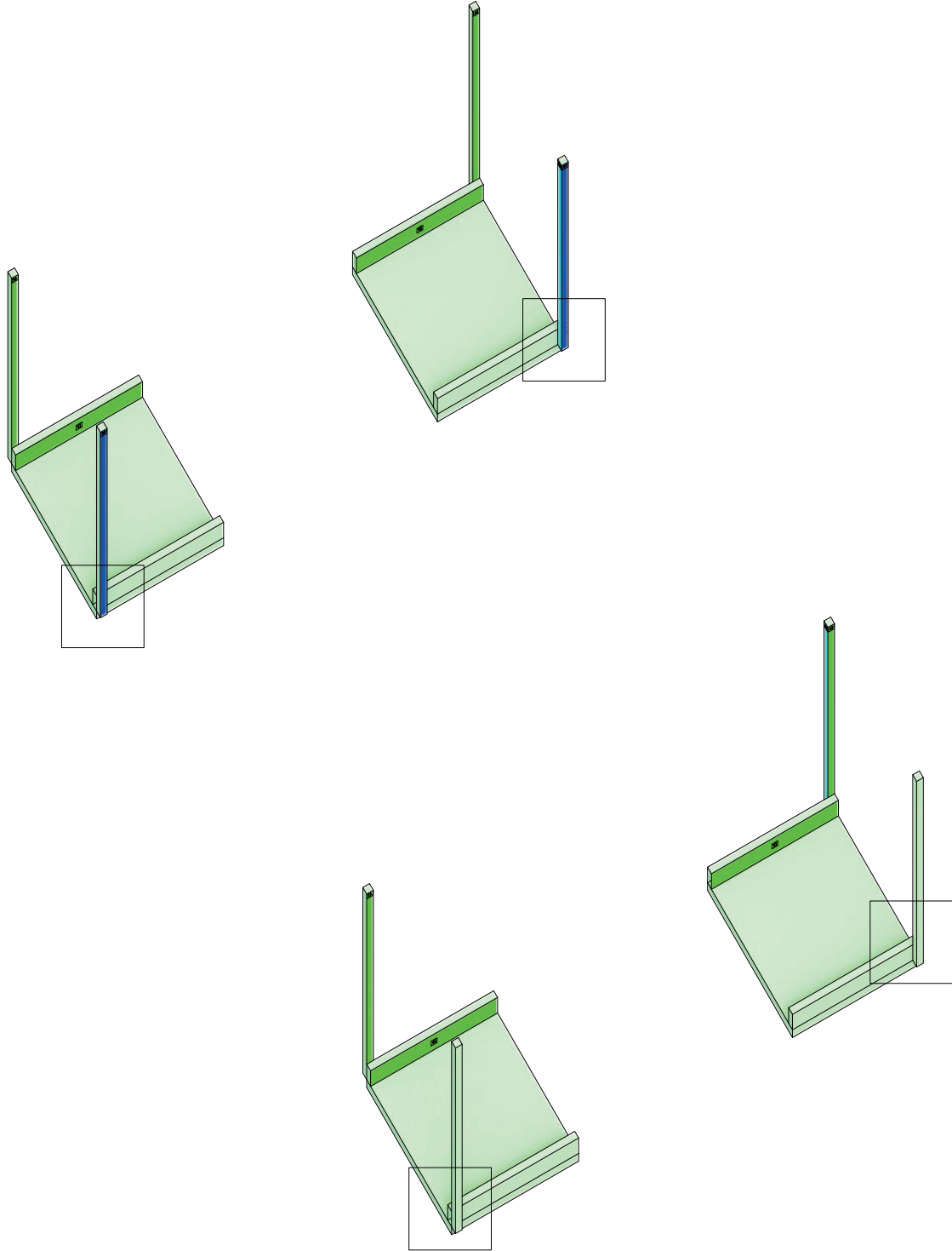
Escritoriolo Despacho. Axonometría. Escala 1:25. 08 Dar vuelta a las ocho bandejas 09 Seleccionar las cuatro bandejas que serán las de la tabla superior de apoyo de la mesa 10 Unir las cuatro bandejas seleccionadas con sus dos respectivas patas
